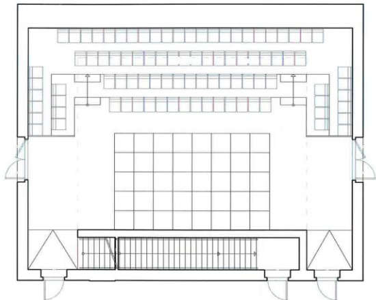
experimentálna sála – alternatíva usporiadania A – pôdorys M1:150
