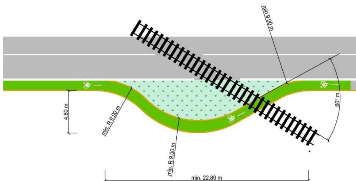
Obrázok 10 - Prejazd cez koľajovú trať odsunutím cyklistického pruhu – optimálne riešenie stavebnou úpravou (Zdroj: TP 085 Navrhovanie cyklistickej infraštruktúry, obrázok 105). (16)
