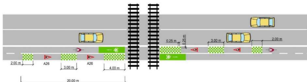
Obrázok 11 - Prejazd CYK cez železničnú trať pomocou dopravného značenia. (16)
