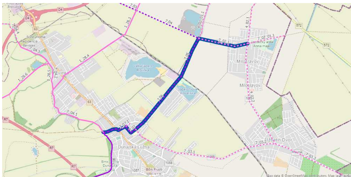
Obr. 4.10 Projekt dopravných cyklistických trás k záchytným parkoviskám pre IDS BSK, Lokalita Nové Košariská – Dunajská Lužná
