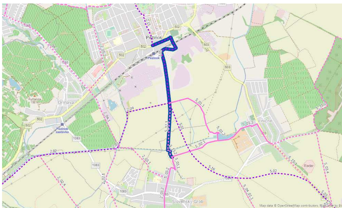
Obr. 4.10 Projekt dopravných cyklistických trás k záchytným parkoviskám pre IDS BSK, Lokalita Pezinok
