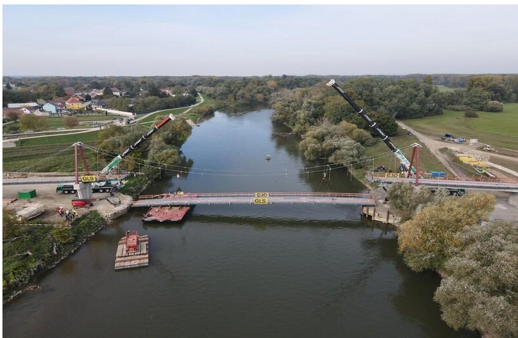
Obrázok č. 1 – Osadenie ocelevej konštrukcie cyklolávky VysoMarch
